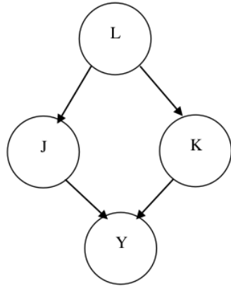
Gambar 2. Contoh analisis bayesian network dengan 4 variabel
