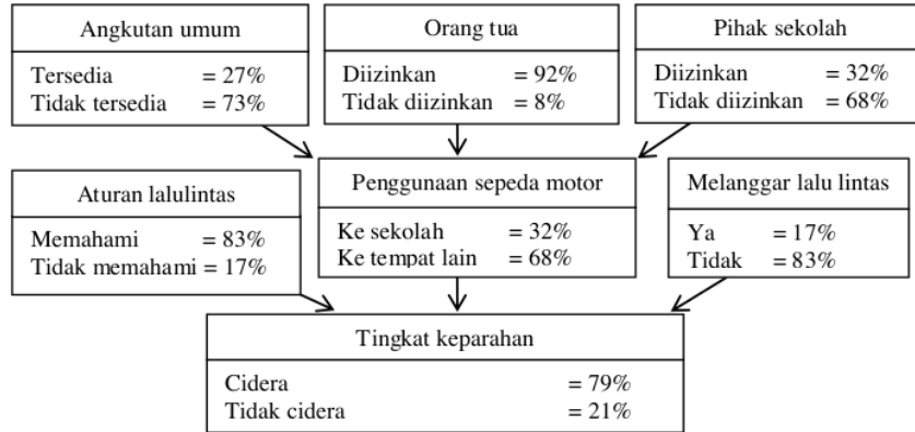
Gambar 3. Model struktur Bayesian network tingkat keparahan kecelakaan
